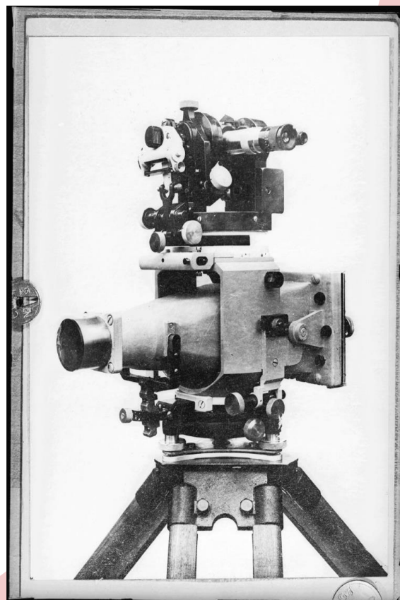
Swisstopo, Wild Phototheodolit, 1926 https://memobase.ch/de/object/blt-001-000398088
